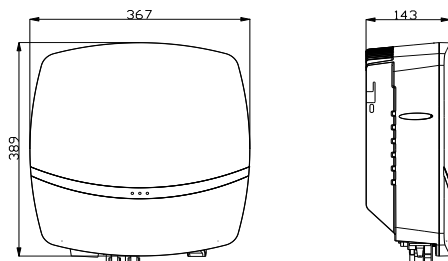
图 3.4 R5-3K/4K/5K/6K-S2, R5-3K/4K/5K/6K-S2-15 外观及尺寸图
