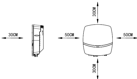
图 4.2 安装间隙
